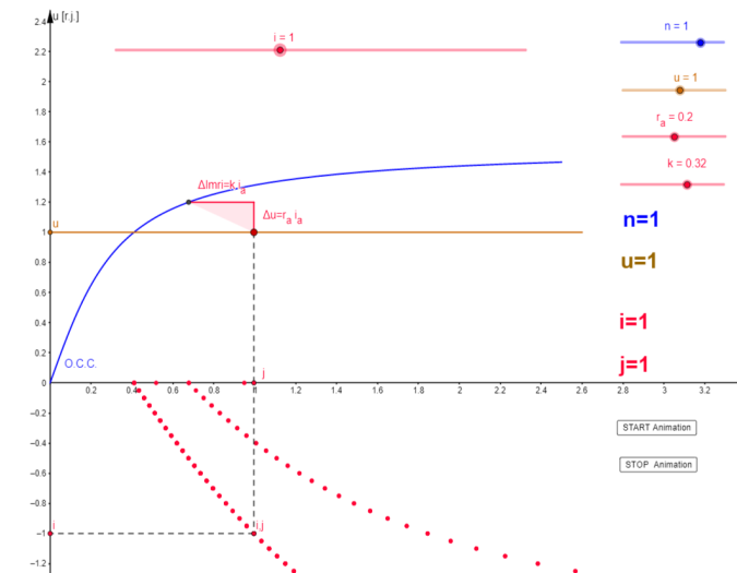
Sl. 7. Karakteristika regulacije generatora jednosmjerne struje sa nezavisnom pobudom [11].
