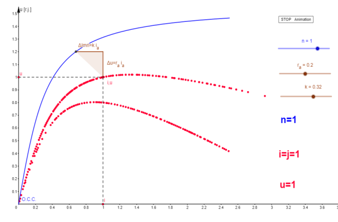
Sl. 10. Spoljna karakteristika generatora jednosmerne struje sa rednom pobudom [14].
